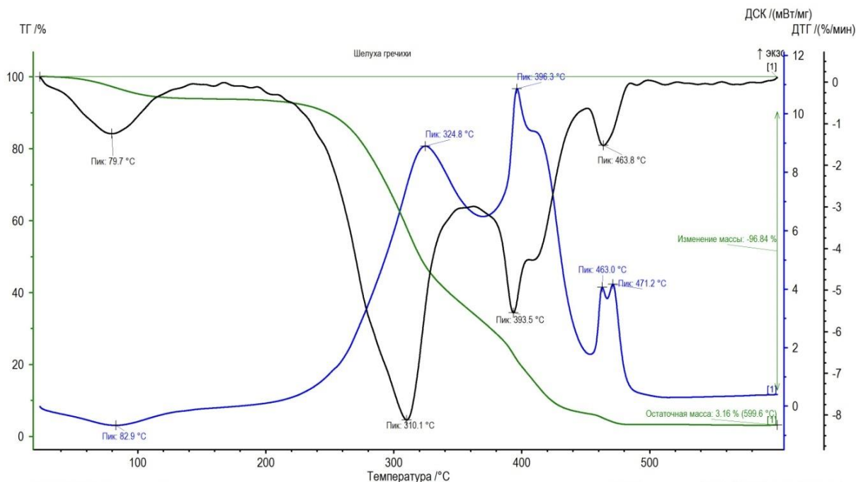
Рис. 4. Кривые ТГ, ДТА и ДСК шелухи гречихи
